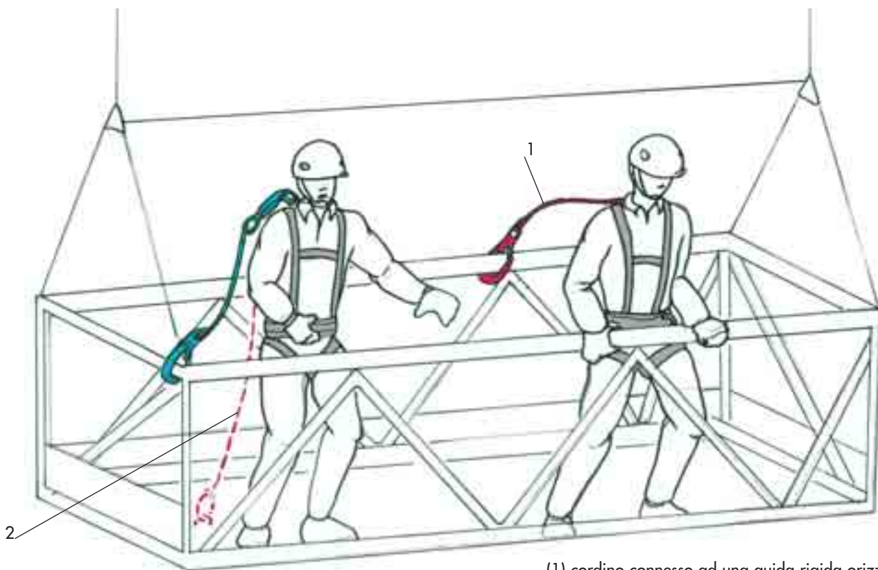
(1) cordino connesso ad una guida rigida orizzontale (2) linea di trattenuta alternativa
