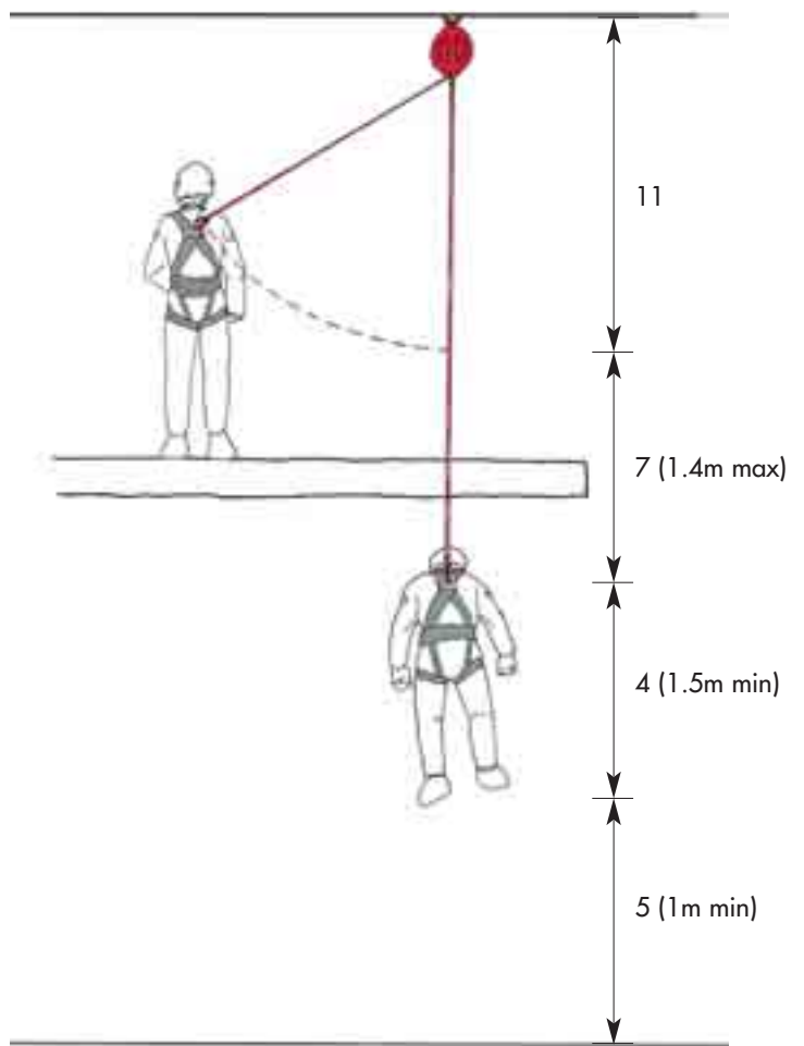
b) Dispositivo retrattile
