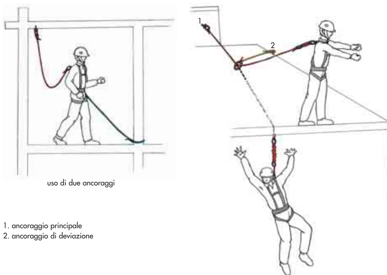
Fig. 39 - Esempi di uso di ancoraggi aggiuntivi
