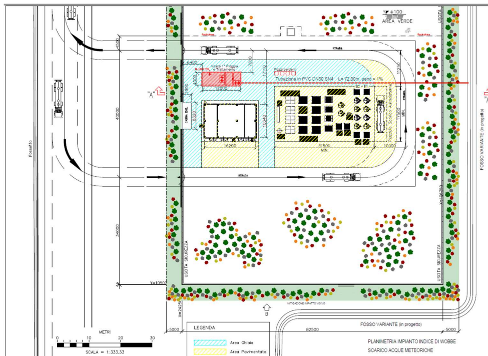
Figura 1 – Planimetria Impianto indice di Wobbe con suddivisione aree pavimentate (in giallo) e in ghiaia (in ciano).
