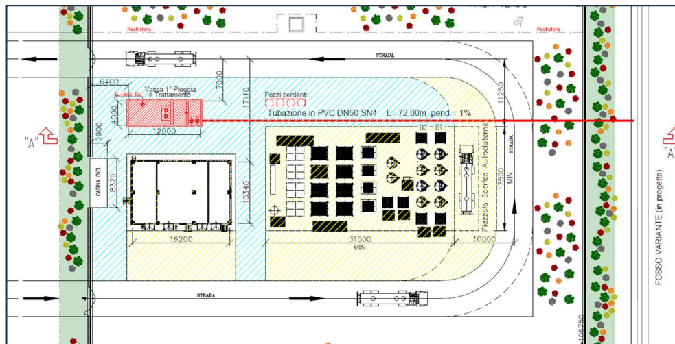
Figura 3 – (in rosso) Sistema smaltimento acque meteoriche di prima e seconda pioggia, previo trattamento
