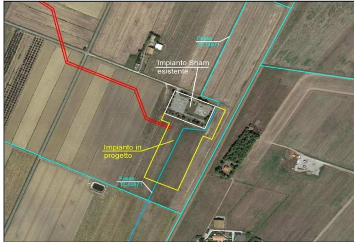
Fig. 2 - Inquadramento planimetrico area di intervento con interferenza fosso T14671: ante operam
