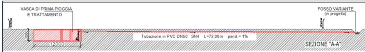
Figura 4 – Sezione A-A: profilo tubazione PVC di scarico al Fosso Variante
