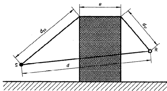
Figura 2 – Geometria della diffrazione singola
